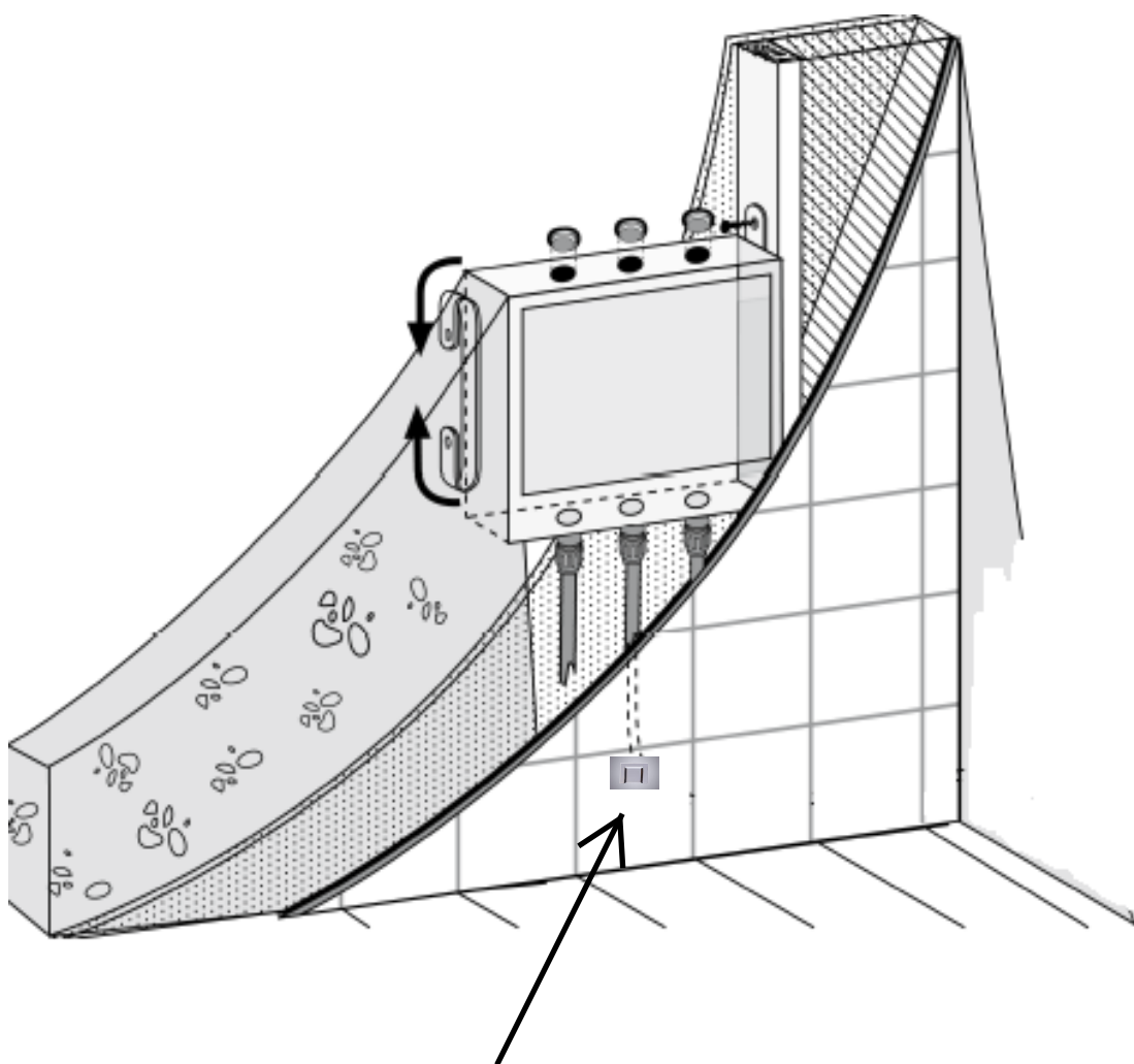
Vuodonilmaisimen ulostulo
