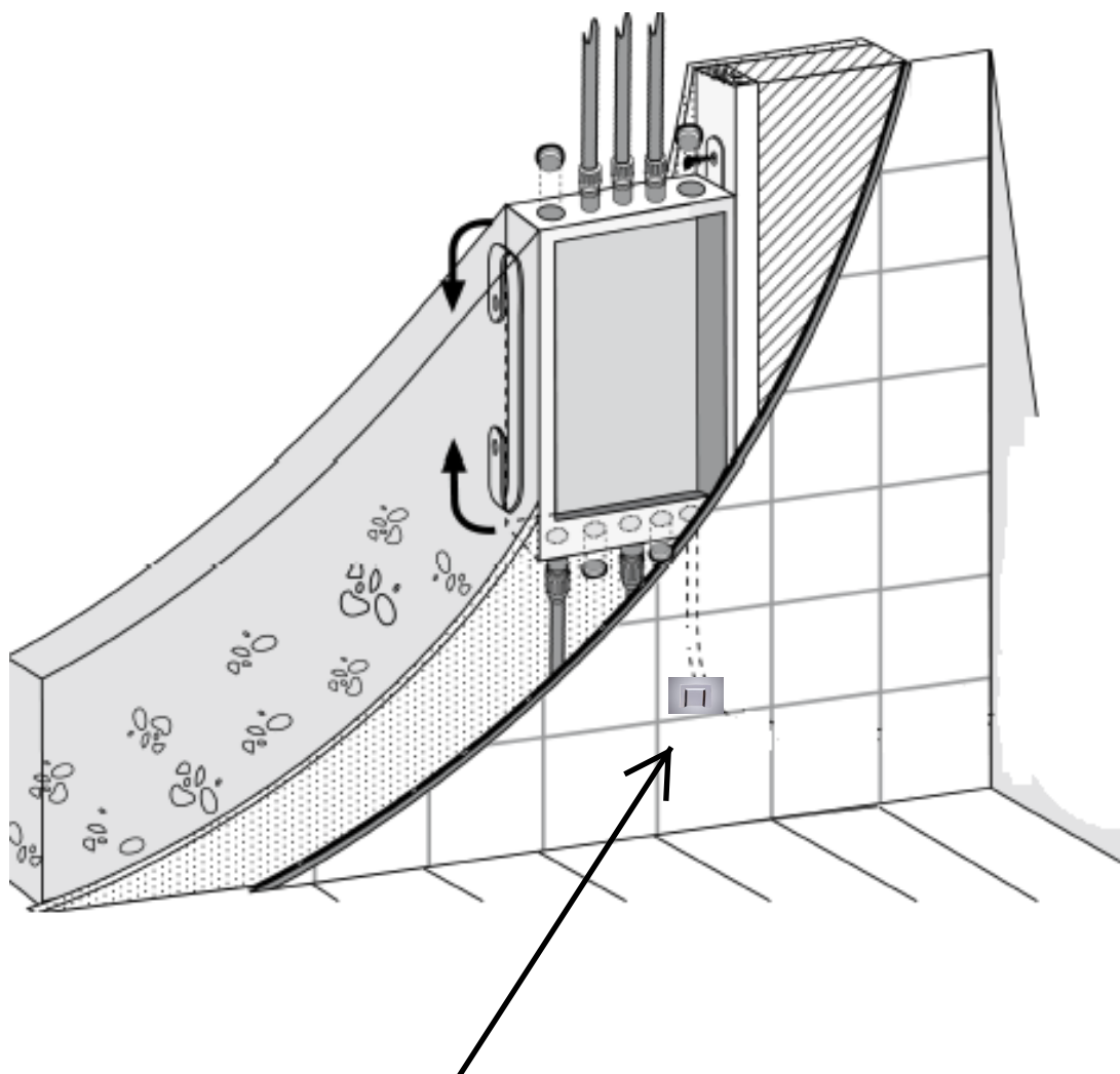
Vuodonilmaisimen ulostulo
