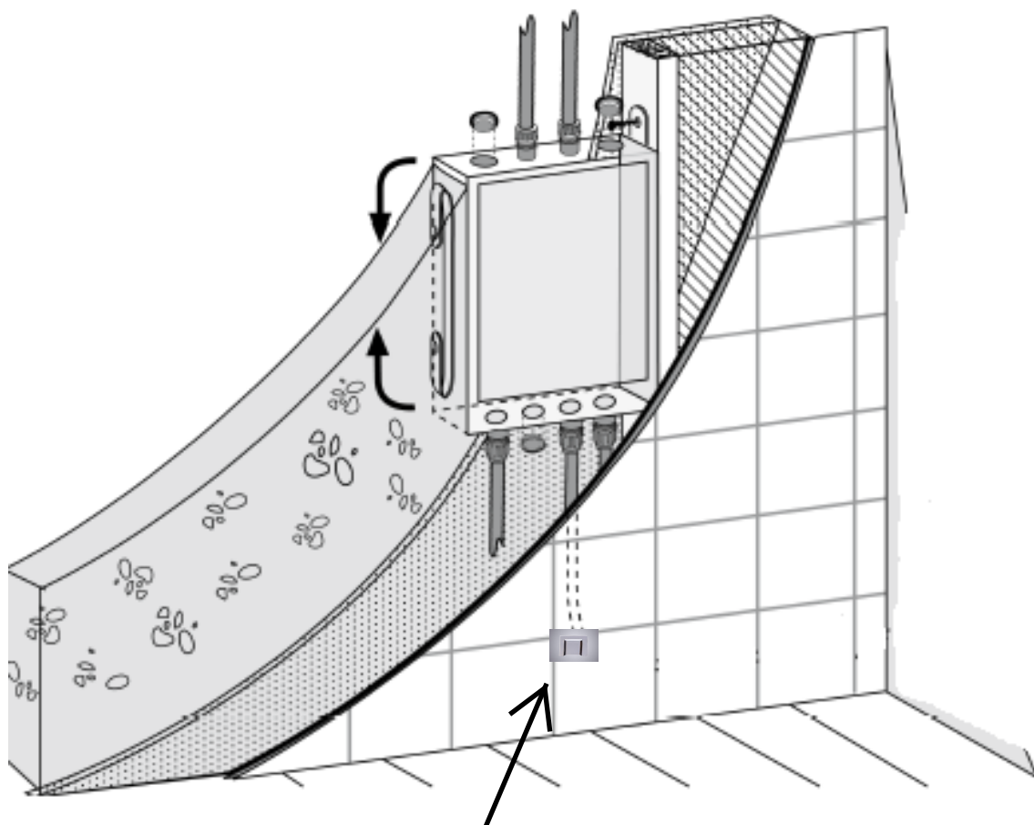
Vuodonilmaisimen ulostulo
